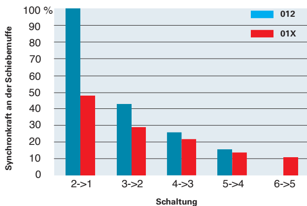
Gegenüberstellung Synchronkraft an der Schiebemuffe
